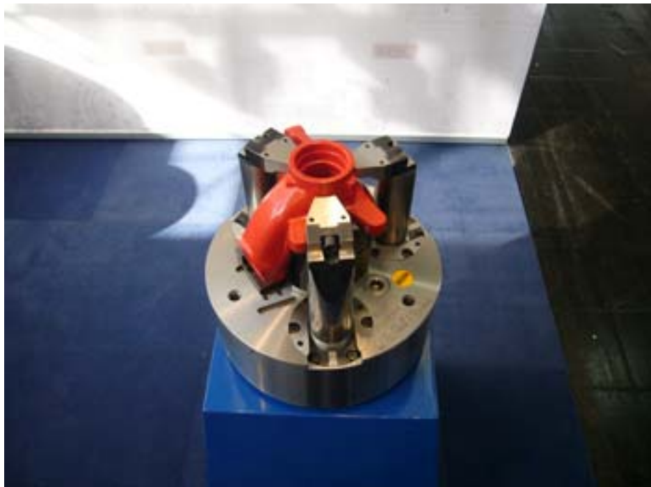
Spannfutter
